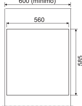
Vista frontal do nicho 600 (mínimo)
