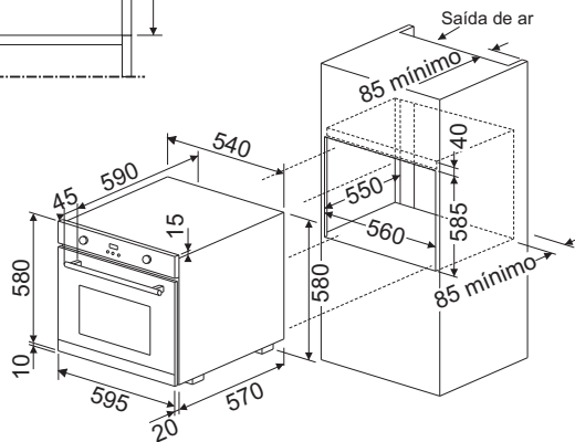
Embutimento em móvel tipo torre
