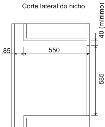
Corte lateral do nicho
